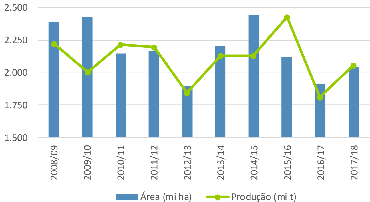
Brasil
