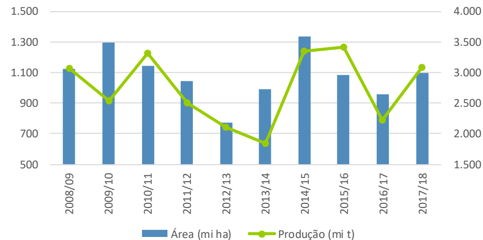
Paraná
