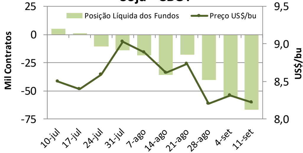
Soja - CBOT
