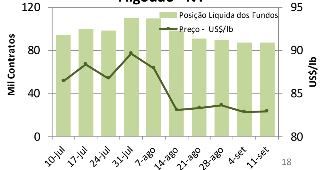
Algodão - NY
