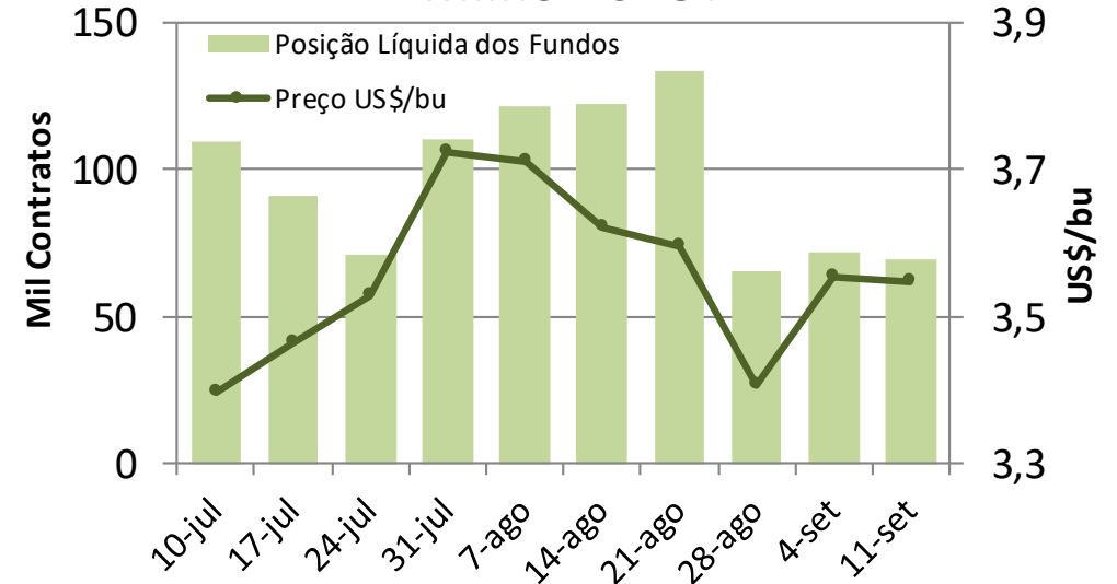
Milho - CBOT
